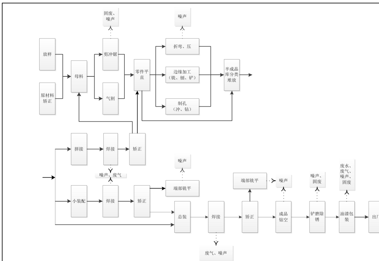
图 2-1 生产工艺流程及产污位置
